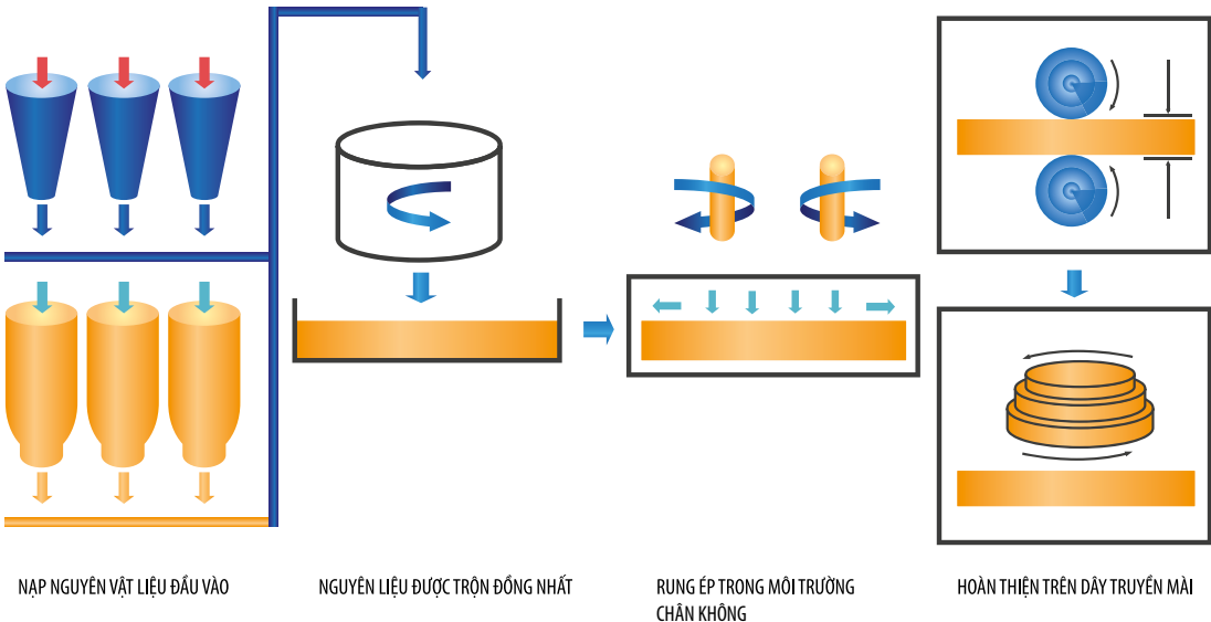
Mô hình công nghệ sản xuất đá nhân tạo
